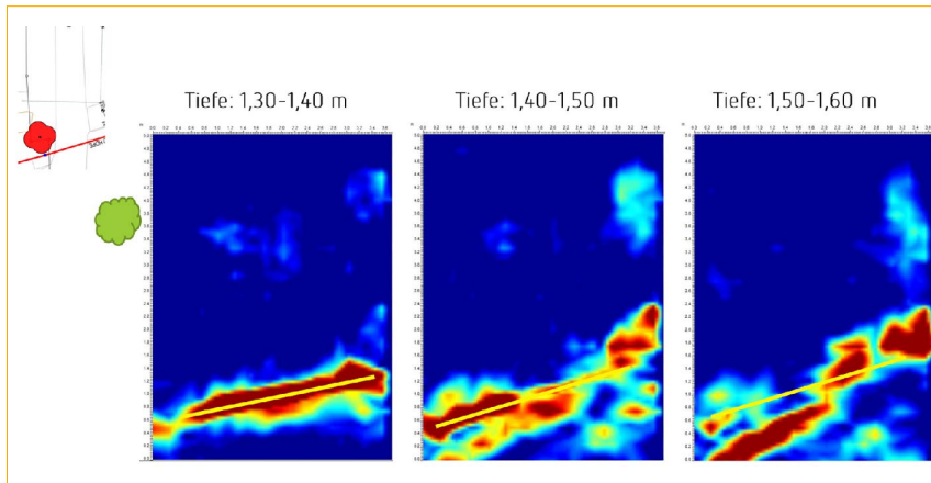
Abb. 09: Leitungsverlauf und Wurzel-Zugschlingen-Nachweis [Quelle: ArborPlan GmbH & Co. KG]
