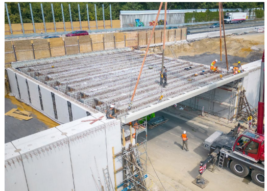
Abb. 04: Montage des Randträgers mit Hybridkappe in Endlage (2. Bauabschnitt), Bauwerk Münsterstraße [Foto: Echthoff GmbH & Co. KG]
