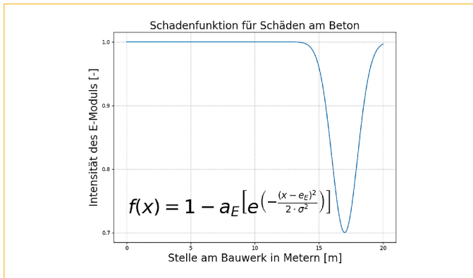
Abb. 04: Beispielhafte Schadenfunktion [Quelle: Lukas Guntermann]
