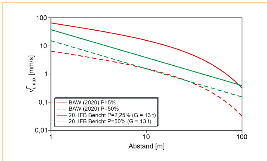
Abb. 02: Prognosegleichungen des 20. IFB-Berichts und der BAW für die maximale Komponente der Fundamentschwinggeschwindigkeit infolge Verdichtung mit Vibrationswalzen [Quelle: Prof. Dr.-Ing. M. Achmus]
