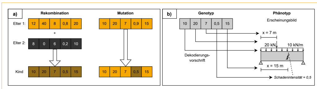
Abb. 02: Überblick über die Funktionsprinzipien Evolutionärer Algorithmen [Quelle: Lukas Guntermann]
