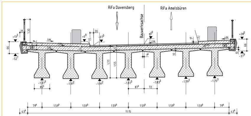
Abb. 06: Regelquerschnitt des Ersatzneubaus Amelsbürener Straße [Quelle: KHP Dortmund]
