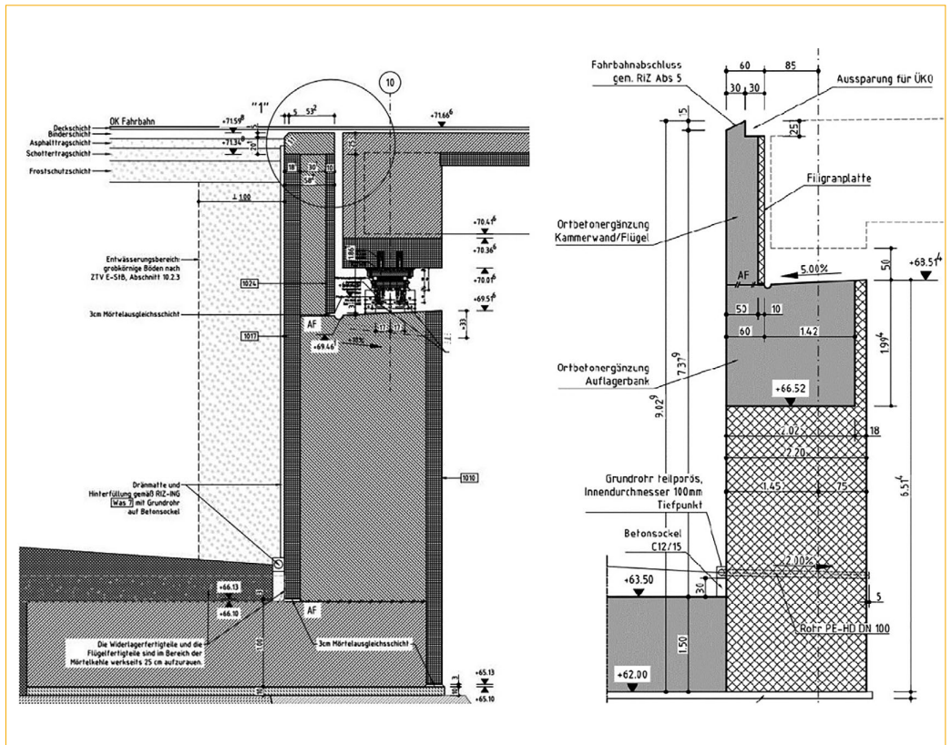
Abb. 01: Ausführungsvarianten der Widerlager in modularer Expressbauweise (Systeme der Unternehmensgruppe Echterhoff), links: Münsterstraße, rechts: Amelsbürener Straße [Quelle: KHP Dortmund/Echterhoff]
