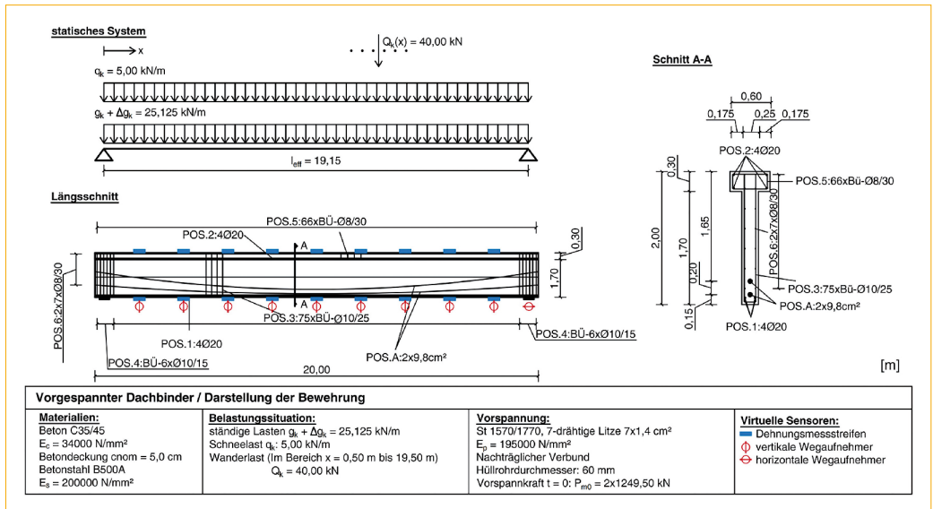
Abb. 08: Validierungsbauwerk – vorgespannter Fertigteildachbinder [Quelle: Lukas Guntermann/ Bjarne Sprenger 9 ]
