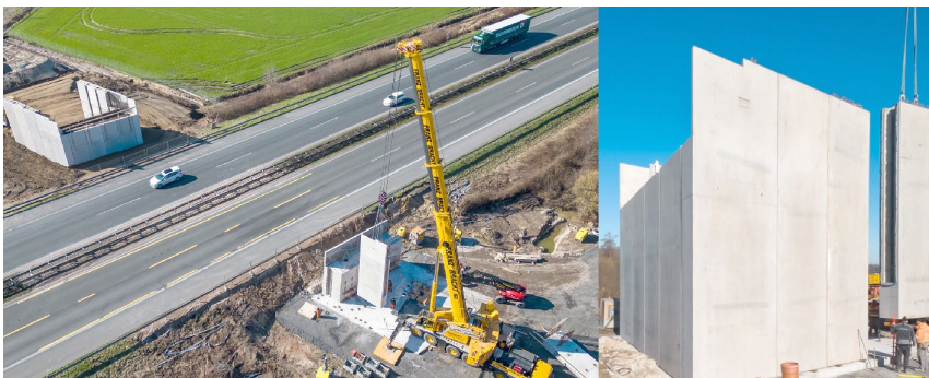
Abb. 07: Aufstellen der modularen Widerlagerelemente, Amelsbürener Straße [Foto: Echthoff GmbH & Co. KG]
