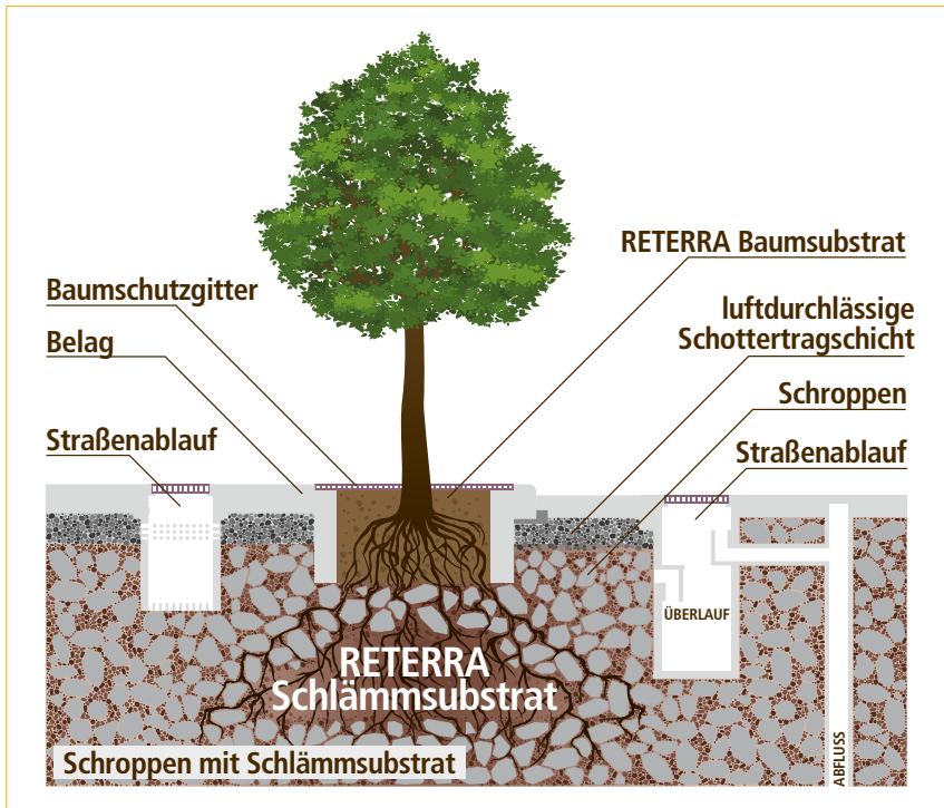
Abb. 01: Schematischer Aufbau einer Baumpflanzgrube mit RETERRA-Schlammsubstrat [Grafik: RETERRA]
