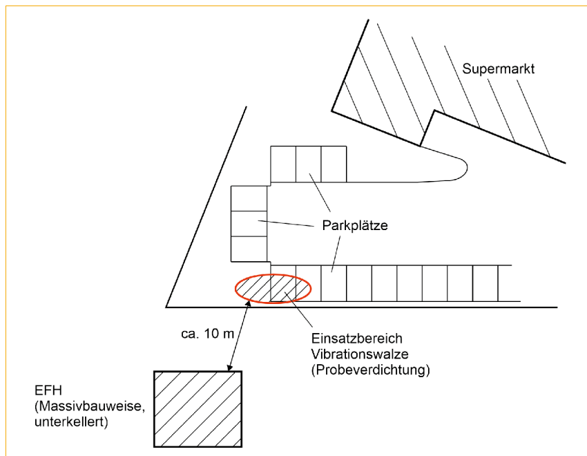
Abb. 01: Beispielskizze der Situation mit dem Abstand zwischen dem Einfamilienhaus und den Parkplätzen [Quelle: Prof. M. Achmus]
