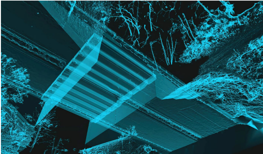
Abb. 08: Geometrische Darstellung mit Röntgen-Effekt der vernetzten Messpunktwolke in der Draufsicht [Quelle: F7 DIGITAL GmbH]
