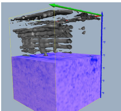
Abb. 07: 3D-Ansicht des gescannten Abschnitts mit »allen« Leitungen [Quelle: ArborPlan GmbH & Co. KG]
