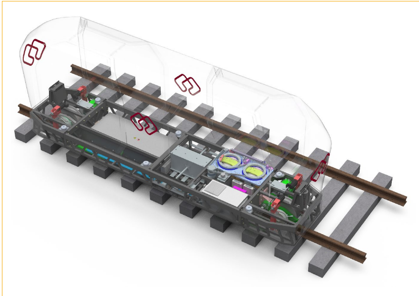
Abb. 02: Das MONOCAB ist eine kreiselstabilisierte Einschienenbahn: Selbstfahrende Kabinen für vier bis sechs Passagiere fahren in beiden Richtungen auf einem Gleis. [Quelle: MONOCAB – TH OWL, M.Sc. Moritz Knitter]
