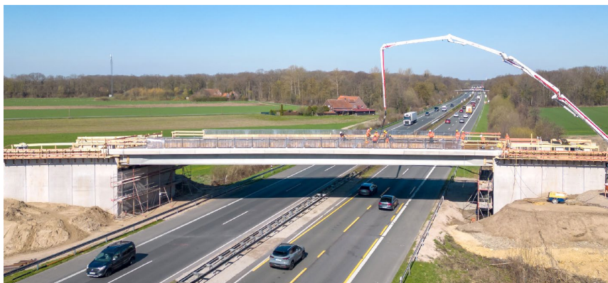
Abb. 11: Betonage der Ortbetonschicht unter laufendem Verkehr, Bauwerk Amelsbürener Straße [Foto: Echterhoff GmbH & Co. KG]
