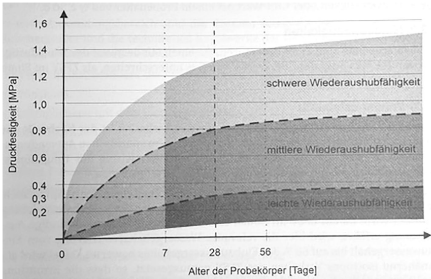
Abb. 02: Schematische Darstellung des Verfestigungsverlaufs 2 [ZFSV]
