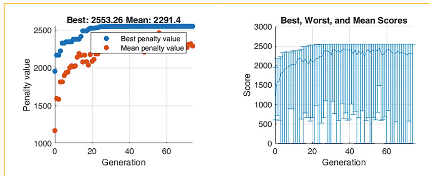
Abb. 10: Beispielhafter MATLAB-Output der Konvergenzergebnisse (Versuch 08 mit N = 75) [Quelle: Lukas Guntermann in MATLAB 12 ]
