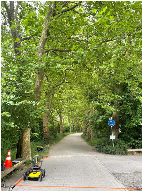
Abb. 08: Messfeld eines Platanenstandorts im Nahbereich der erdverlegten Leitung [Foto: ArborPlan GmbH & Co. KG]
