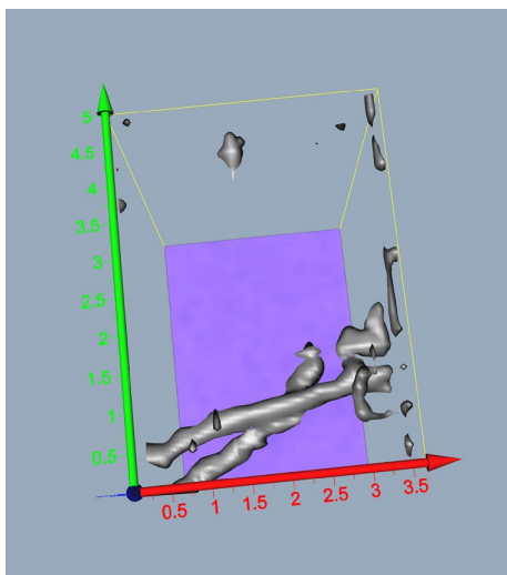
Abb. 10: 3D-Nachweis der Wurzel-Leitungs-Interaktion [Quelle: ArborPlan GmbH & Co. KG]
