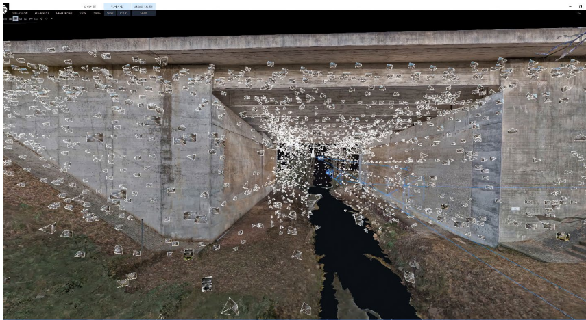
Abb. 07: Darstellung der räumlichen Anordnung der einzelnen rund 5400 Auslösemomente der Kamerapositionen [Quelle: F7 DIGITAL GmbH]
