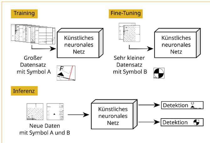
Abb. 02: Schema der beiden evaluierten FSD-Methoden Brute-Force-Baseline (BFB) und Two-Step-Fine-Tuning-Approach (TFA) [Quelle: Ruhr-Universität Bochum]
