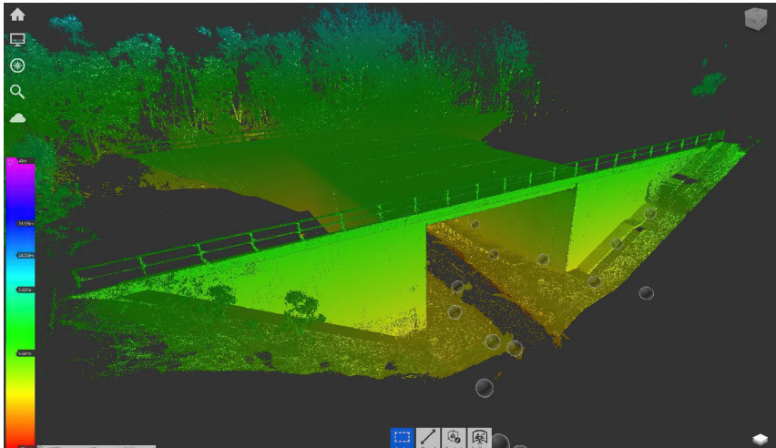
Abb. 05: Darstellung der 3D-Messpunktwolke ausschließlich aus den terrestrischen Laserscans [Quelle: F7 DIGITAL GmbH]
