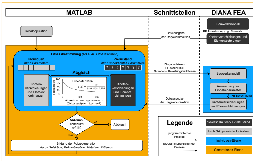
Abb. 06: Konzept der Programmierung des Genetischen Algorithmus [Quelle: Lukas Guntermann, angelehnt an Guntermann/Sprenger(2024) 8 ]
