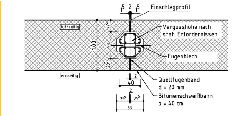
Abb. 02: Planauszug zur wasserdichten Betonplombe zwischen den Flügelwandelementen (System der Unternehmensgruppe Echterhoff), hier: Ausführung Amelsbürener Straße [Quelle: KHP Dortmund/Echterhoff]
