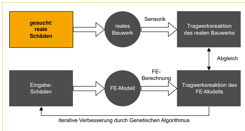
Abb. 01: Schematische Darstellung der Strukturidentifikation durch FE-Model-Updating [Quelle: Lukas Guntermann]
