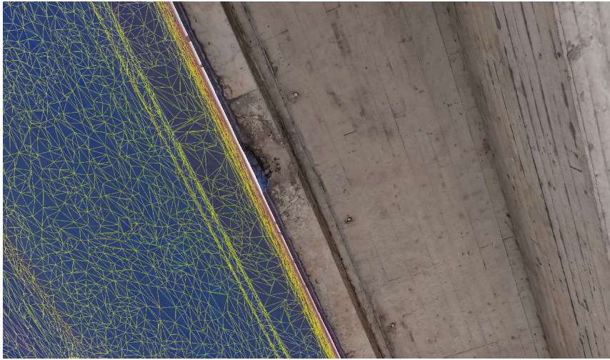
Abb. 09: Visualisierung aus dem vernetzten 3D-Ergebnis mit Fototexturen und einer detektierten Schadstelle [Quelle: F7 DIGITAL GmbH]
